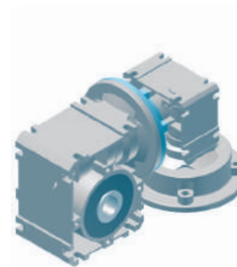
Конструктивное исполнение U8
