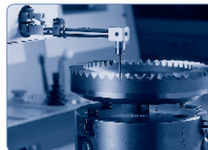
Компьютерное измерение профиля зуба шестерни
