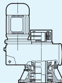
SK ..82 AFSH VL2 mm ⇒ D117 SK ..82 AFSH VL3
